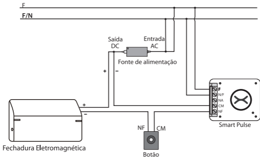
Exemplo de instalação em uma Fechadura Eletromagnética
